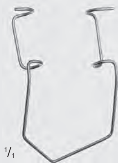
H-1049 Kratz-Barraquer Lidsperrer, groß, starker Draht Eye speculum, large, heavy wire Blefaróstato, grande, alambre fuerte Blépharostat, grand, ressort fort
