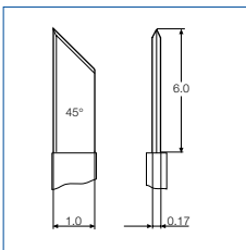
H-1393/2 45° Doppelschneidkante 45° double cutting edge 45° filo doble 45° double tranchant
