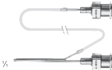
H-5380 O'Gawa Saug- und Spülkanüle, 0,9 x 32 mm, 20 ga Irrigation-Aspiration Cannula, 0,9 x 32 mm, 20 ga Cánula para Irrigación y Aspiración, 0,9 x 32 mm, 20 ga Canule pour aspiration et irrigation 0,9 x 32 mm, 20 ga
